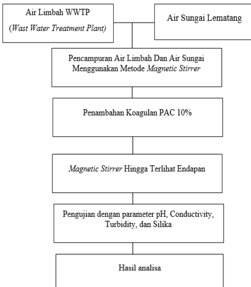
Gambar 2. Skema Penelitian Penentuan Kadar Air Limbah Di Campur Dengan Air Sungai pH
