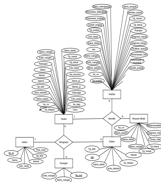
Gambar 5. ERD Sistem Informasi Kelengkapan
