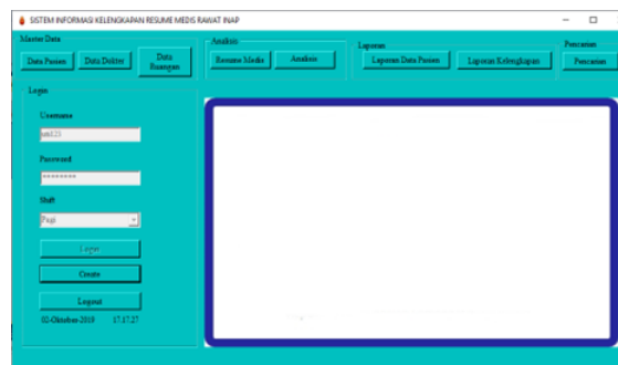
Gambar 10. Menu Utama
