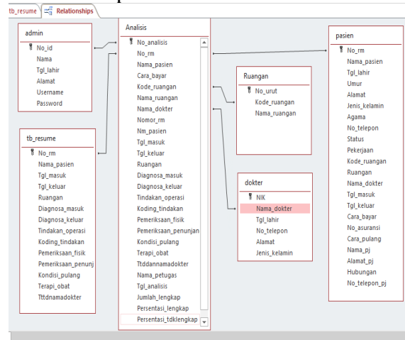
Gambar 6. Relasi Tabel
