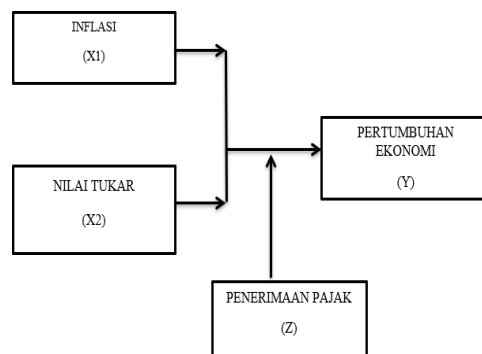
Gambar 1. Kerangka Konseptual
